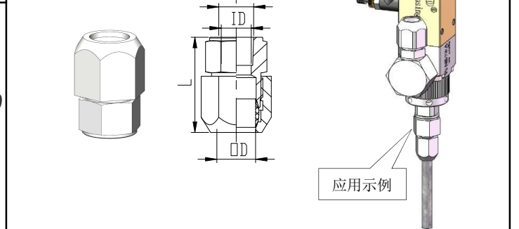
“L”型 外螺纹锁管接头
