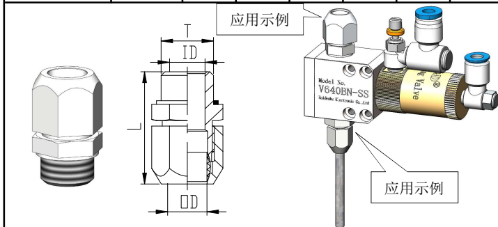
“L”型 外螺纹锁管接头
